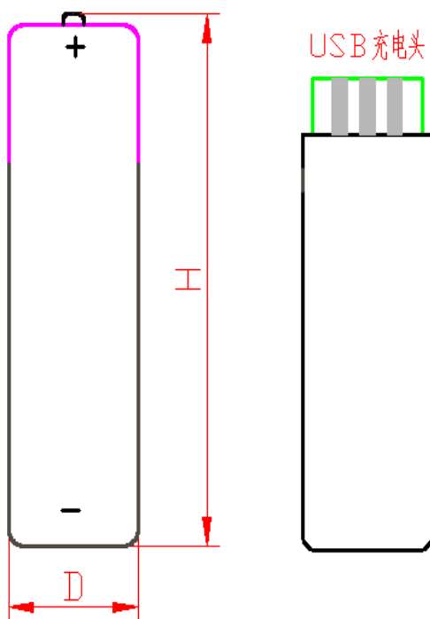
(产品外形尺寸图)
